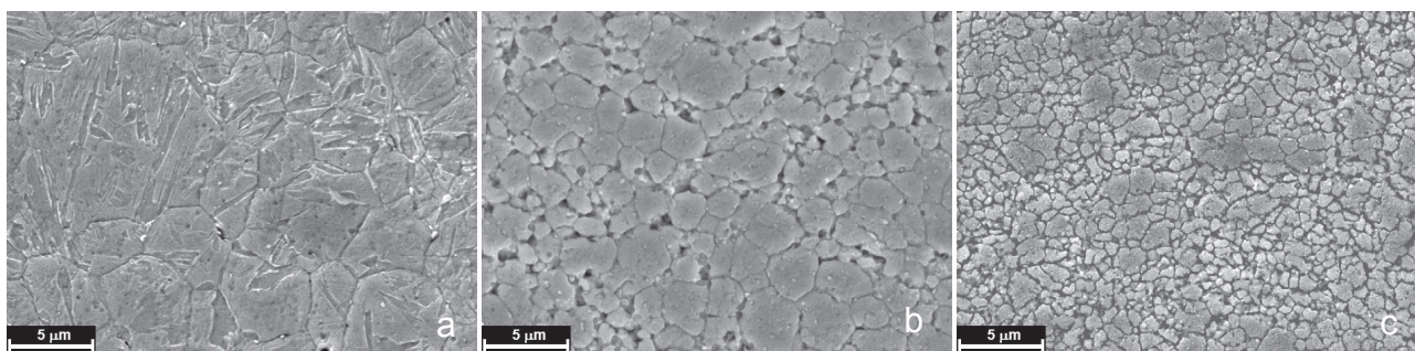
Fig. 7 - Immagini SEM della microstruttura dei campioni sinterizzati da polvere atomizzata (a) e da polvere macina per 200min (b) e 1000min (c).
