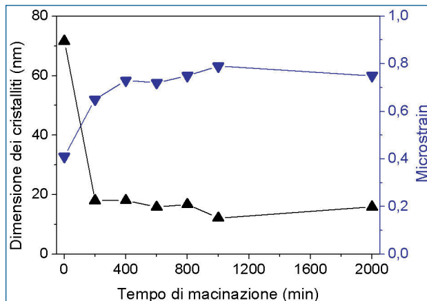
Fig. 4: Dimensione dei cristalliti e microstrain in funzione del tempo di macinazione.
