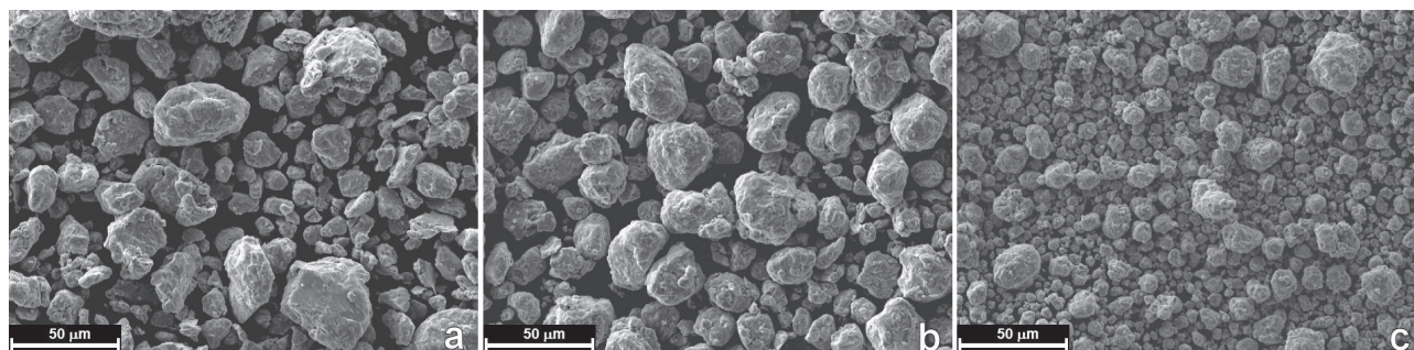
Fig. 2 - Immagini al SEM della polvere di AISI H13 macinata per 200min (a), 400min (b) e 1000min (c).
