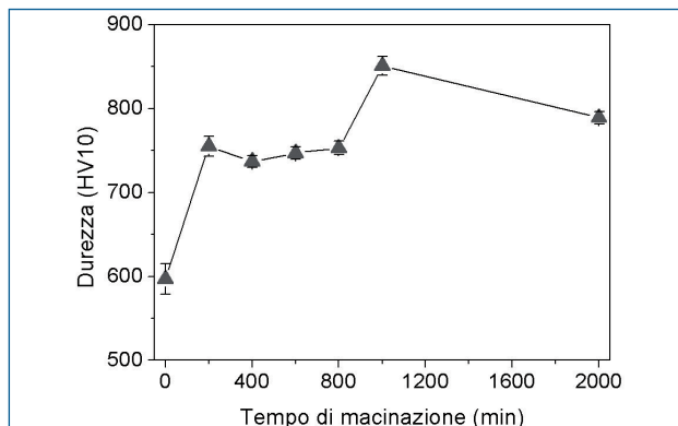
Fig. 9: Durezza dei campioni sinterizzati in funzione del tempo di macinazione.
