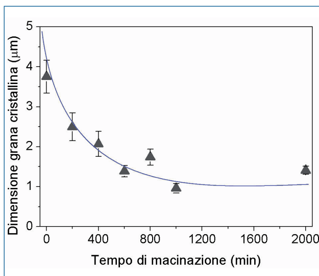
Fig. 8: Dimensione della grana cristallina dei campioni SPS in funzione del tempo di macinazione.
