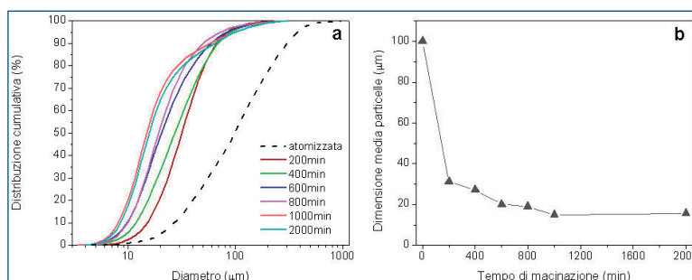
Fig. 3 - Curve cumulative della distribuzione granulometrica (a) e dimensione media delle polveri (b) in funzione del tempo di macinazione.
