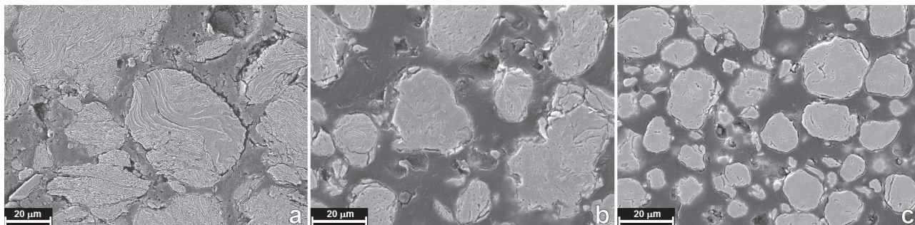
Fig. 6 - Immagini SEM della microstruttura delle polveri di AISI H13 macinate per 200min (a), 400min (b) e 2000min (c).
