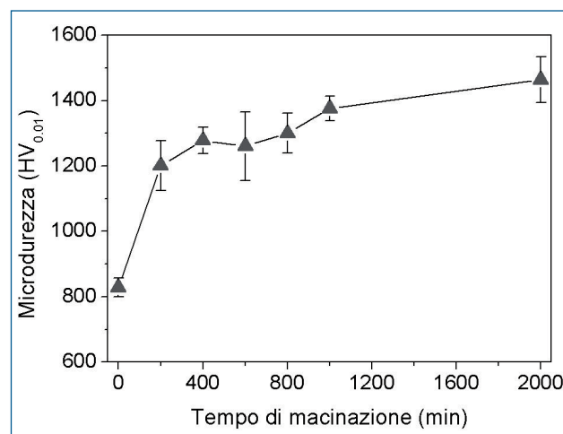
Fig. 5: Microdurezza (HV 0.01 ) delle polveri in funzione del tempo di macinazione.
