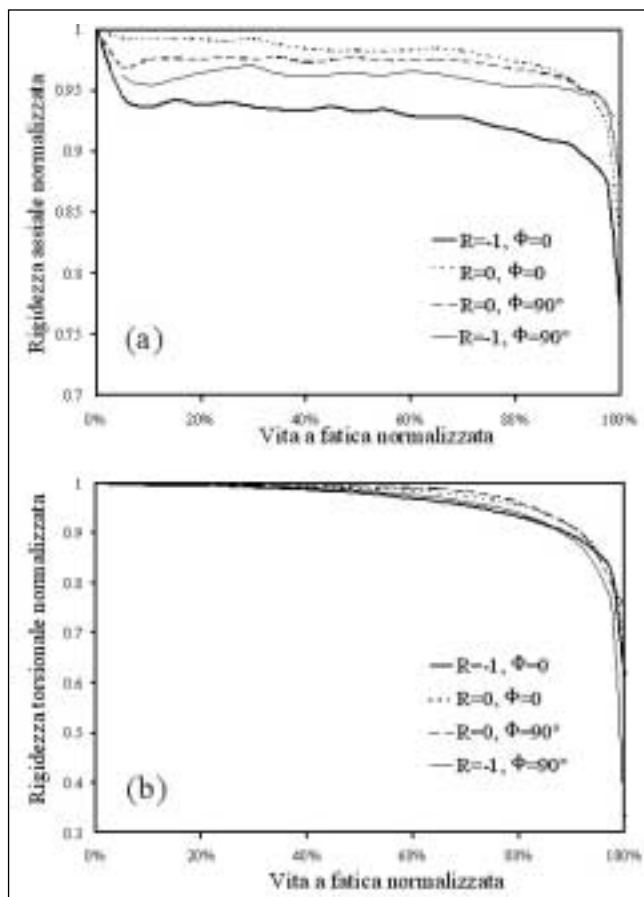
Fig. 10 – Curve di rigidezza assiali (a) e torsionali (b) per i provini intagliati soggetti a fatica multiassiale.
