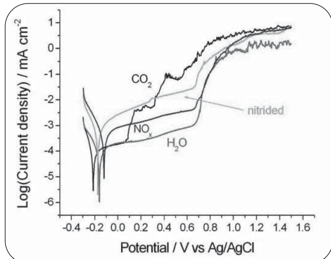
Fig. 4 Curve potenziodinamiche per i quattro trattamenti studiati. PD curves of tested specimens.
