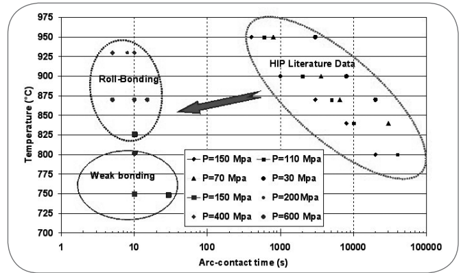
Fig. 6 Grafico dei parametri di processo. Processing parameters.
