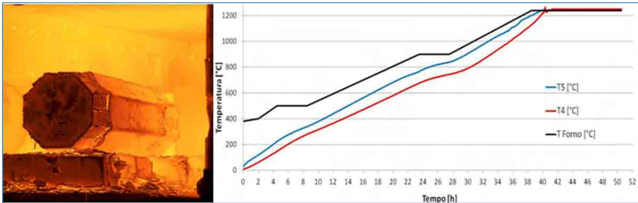
Fig. 8 - Temperatura del forno ( T_{\text{Forno}} [^{\circ}\text{C}] ), della termocoppia in superficie ( T5 [^{\circ}\text{C}] ) e della termocoppia a cuore ( T4 [^{\circ}\text{C}] ) in funzione del tempo [h] per il 26NiCrMoV11.5.
