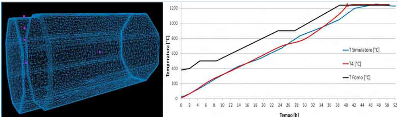
Fig. 9 - Temperatura del forno implementata nel simulatore ( T_{\text{Forno}} [^{\circ}\text{C}] ), della termocoppia a cuore reale ( T4 [^{\circ}\text{C}] ) e della termocoppia a cuore simulata ( T_{\text{Simulatore}} [^{\circ}\text{C}] ) in funzione del tempo [s] per il 26NiCrMoV11.5.
