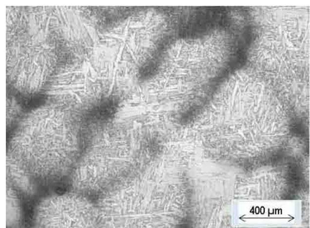
Fig. 4 - Micrografia lingotto poligonale 26NiCrMoV11.5 in posizione centrale
